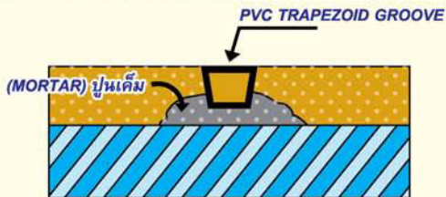
ภาพประกอบ : ลักษณะการติดตั้ง สีเหลี่ยมคางหมู
